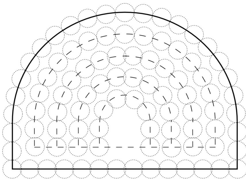
Рис. 1. Схема расположения вспомогательных и оконтуривающих шпуров по забою выработки с учетом влияния вновь создаваемой открытой поверхности. Пунктирными окружностями показаны расчетные радиусы разрушения породного массива без учета влияния открытой поверхности
